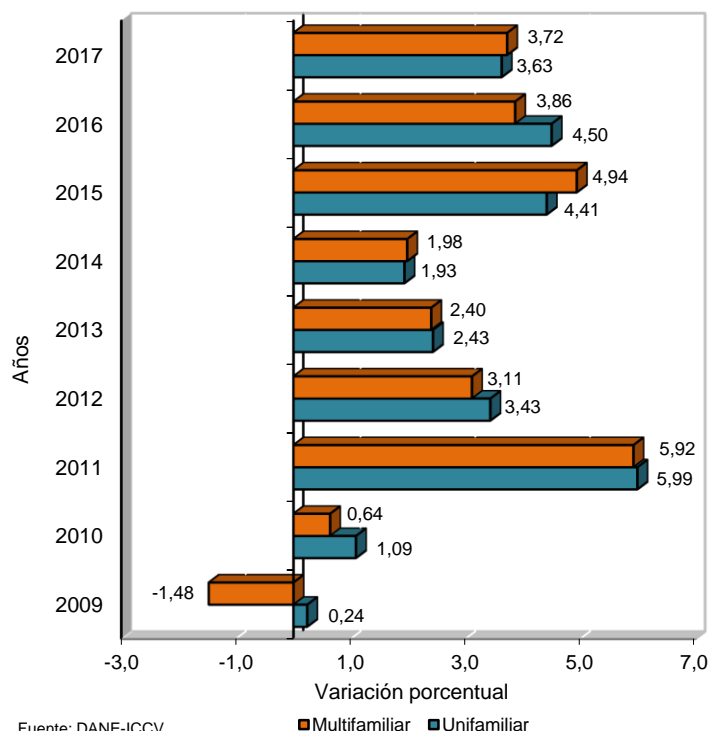
Grafico 4. ICCV. Variación doce meses, por tipo de vivienda Septiembre (2009 - 2017)
